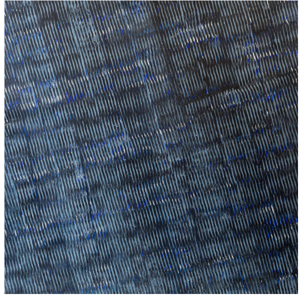
Flysch
